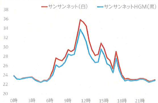
2022年8月14日 サンサンネットHGM温度試験(℃)
